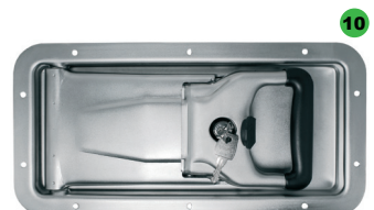
Eingebautes Thiriet-Schloss \varnothing 16 mm.
