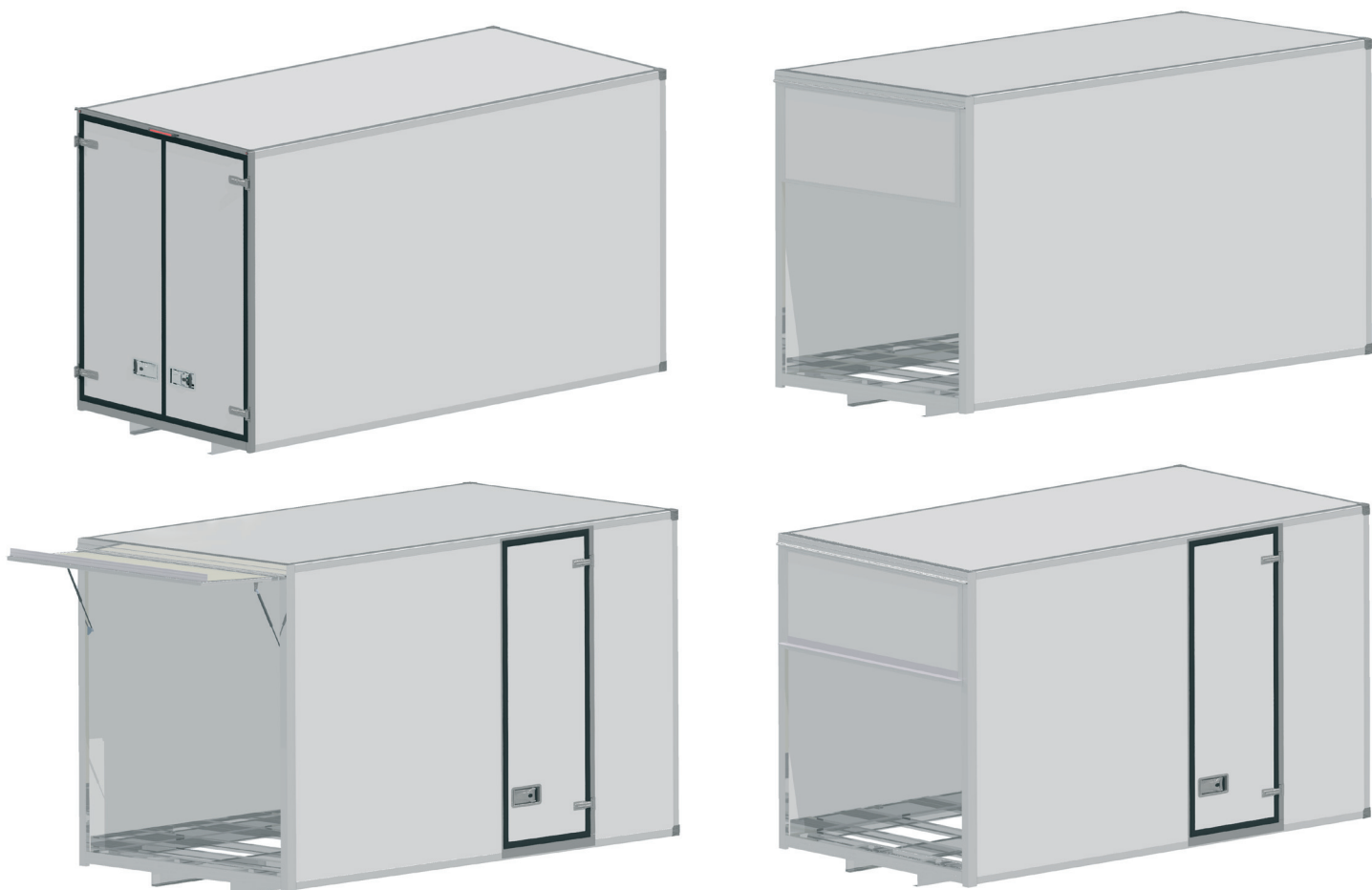
Variante „8 Palettenstellplätze“ ohne Seitentür – Gewicht ab 350 kg.
